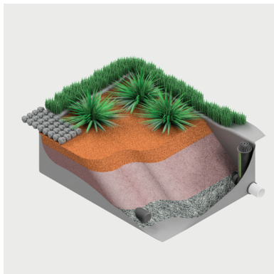
Biofiltre EcoStream™ (Géomembrane)
