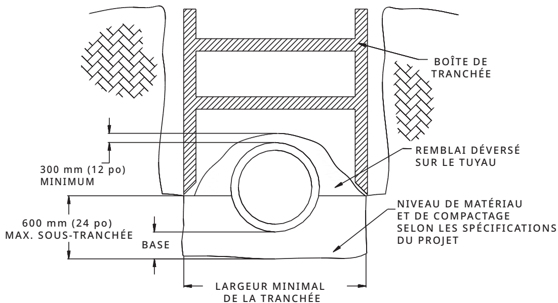
Figure 2 : Installation de sous-tranchée
