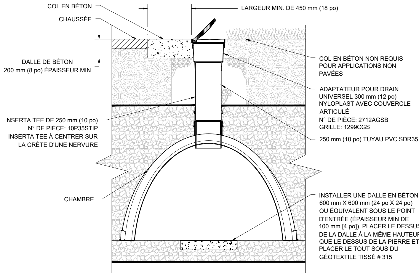
DÉTAIL POINT D'INSPECTION 250 mm (10 po) SERVANT D'ENTRÉE PAS À L'ÉCHELLE
