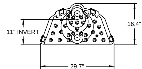
POSILOCK ENDPLATE
