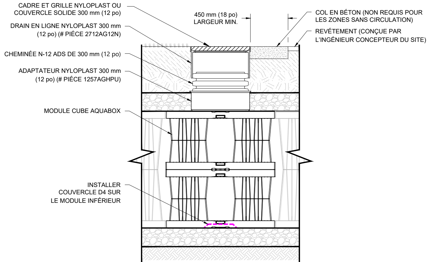
DÉTAIL DU POINT D'INSPECTION AQUABOX NTS
