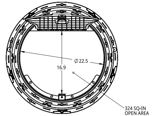
EZSET RISER
