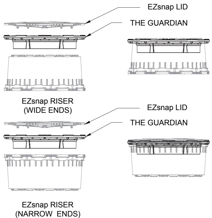
EZSNAP RISER
